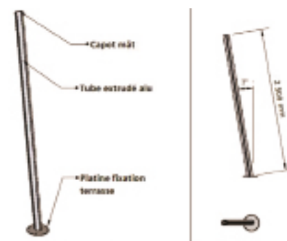
Mât sur plot béton
