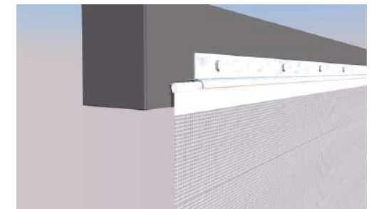
Fixation par clip ou câble
