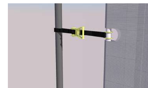
Tension par sangles cliquet
